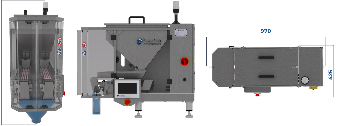
Ön Görünüş
